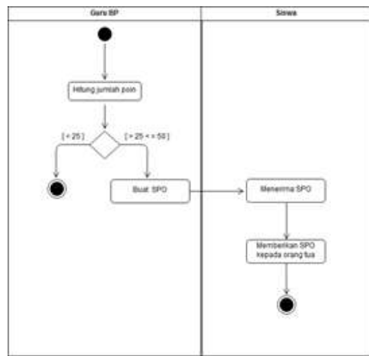
Gambar 3. Activity Diagram Pembuatan Surat Panggilan Orangtua
