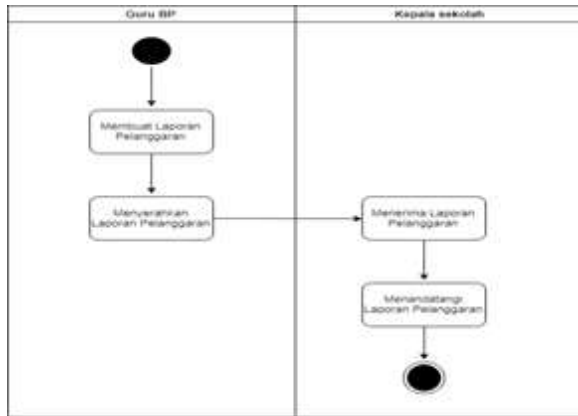
Gambar 5. Activity Diagram Proses Pembuatan Laporan Poin Pelanggaran
