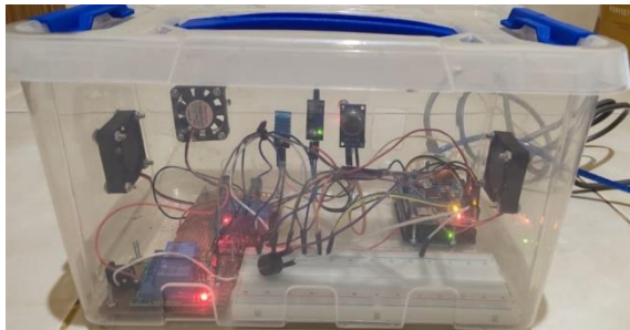
Gambar 3. Rangkaian Alat pada Box Simulasi
