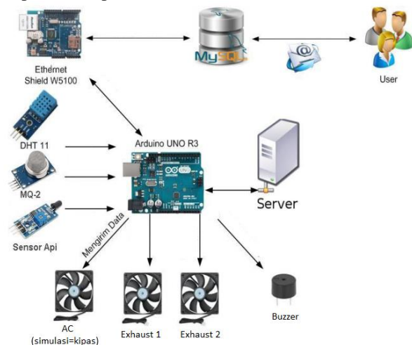
Gambar 2. Arsitektur Sistem
